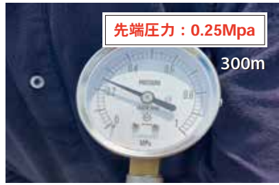
圧力測定器による測定
